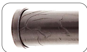
フローマーク(しわ模様)
